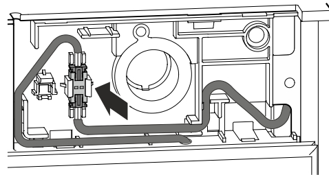
31. Steckerverbindung in die Halterung einrasten. Kabel wie angezeigt verlegen.
