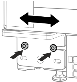
27. Schrauben lösen und Scharnierwinkel nach rechts oder links verschieben.
