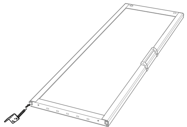
23. Scharnierwinkel, wie in der Abbildung gezeigt, einsetzen und festhalten.
