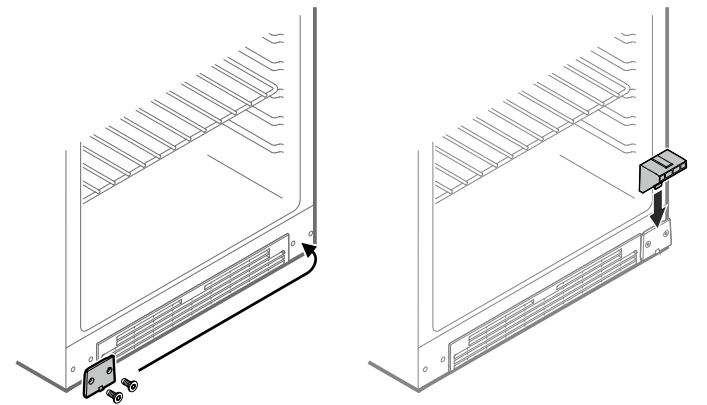
21. Abdeckplatte auf Gegenseite umsetzen.
