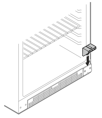
22. Transportsicherung aufsetzen.
