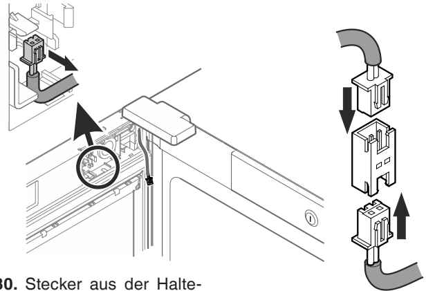
Beide Stecker mit der Steckerkupplung verbinden.
