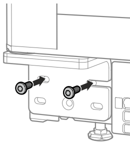
26. Scharnierwinkel anschrauben.
