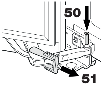
50. Bolzen einsetzen. 51. Roten Sicherungsbügel abnehmen.
